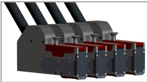
Jet-E .HP22 bis zu 4 Köpfe je 22mm
